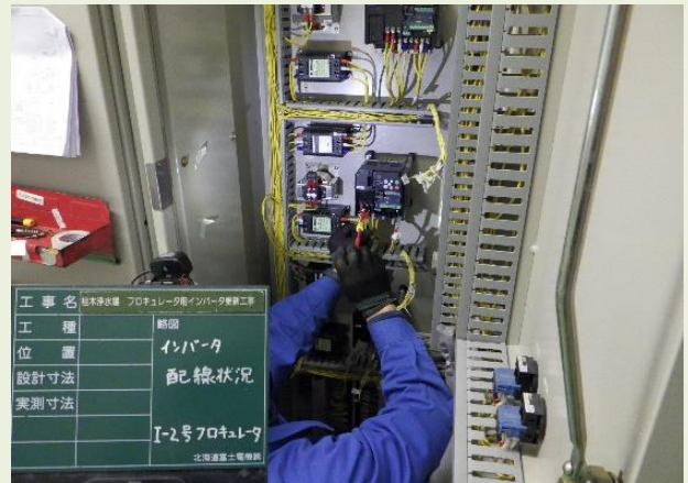
桂木浄水場フロキュレータ用インバータ更新工事
