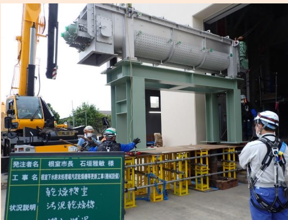
根室下水終末処理場汚泥乾燥機等更新工事
