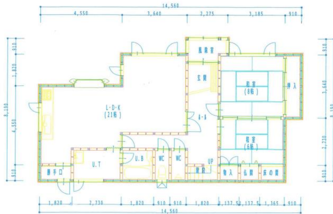
1F 平面図
