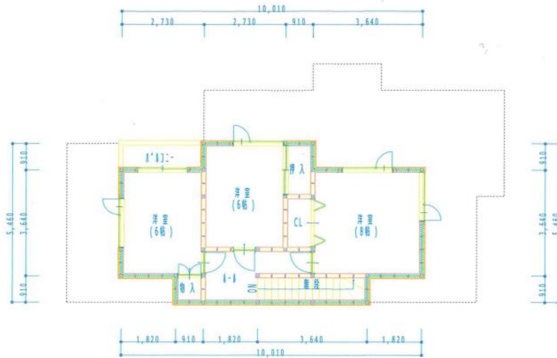
2F 平面図
