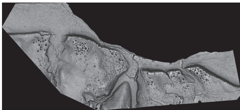
ドローンレーザー測量から 得られた立体図（別当賀川口）
